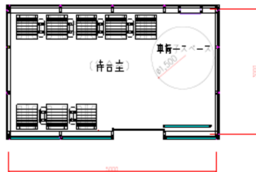
待合室平面図(イメージ)
